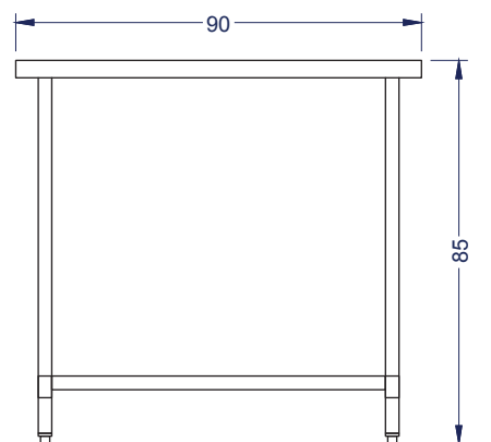
Vista Elevación
