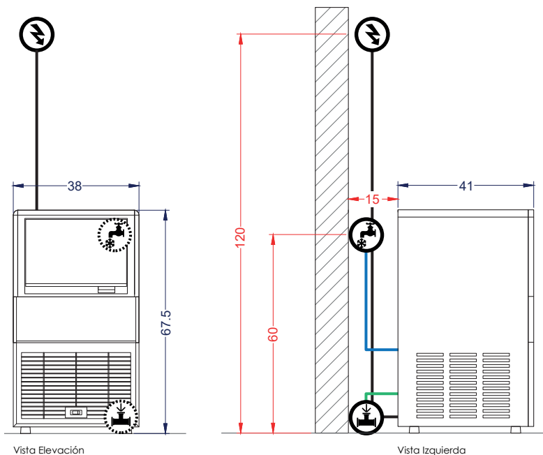
Vista Elevación
