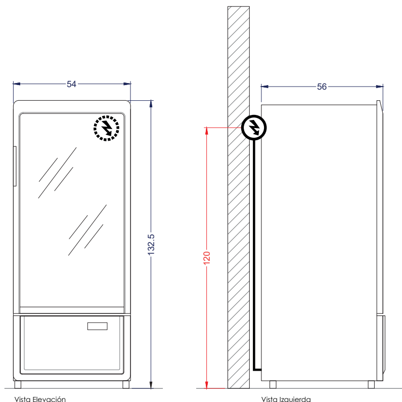
Vista Elevación
