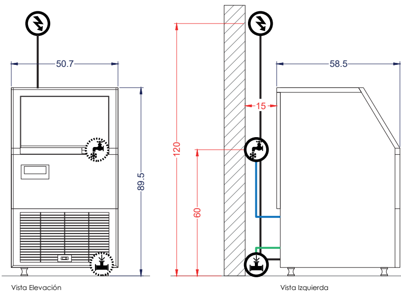
Vista Elevación
