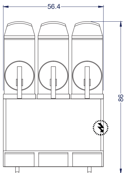
Vista Elevación
