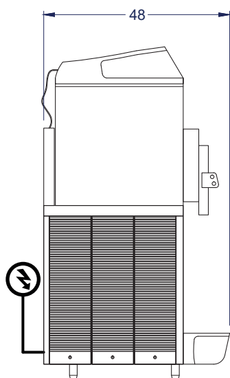
Vista Izquierda
