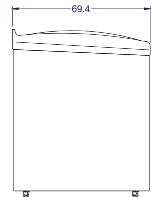
Vista Izquierda
