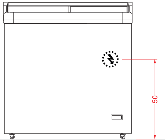
Vista Elevación
