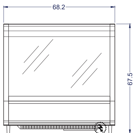
Vista Elevación
