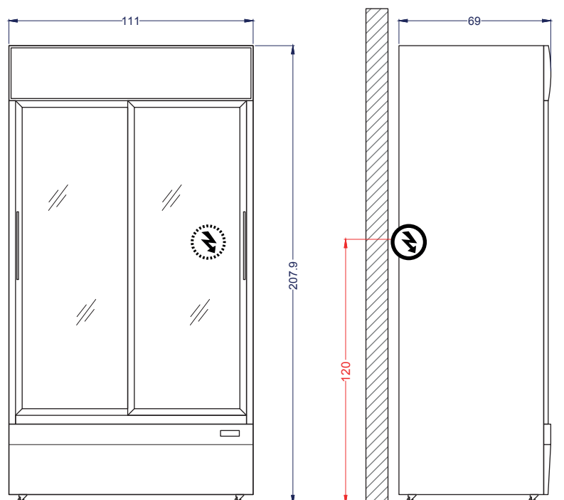
Vista Elevación
