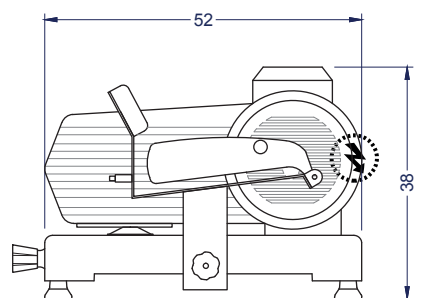
Vista Elevación
